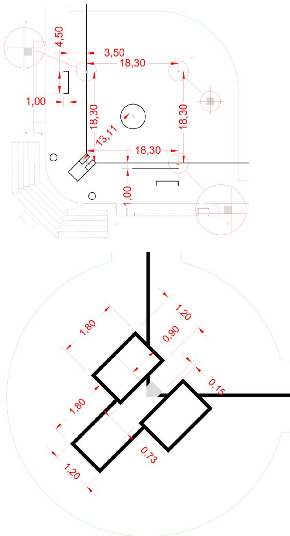
Afbeelding 7 Afmetingen softbalveld
